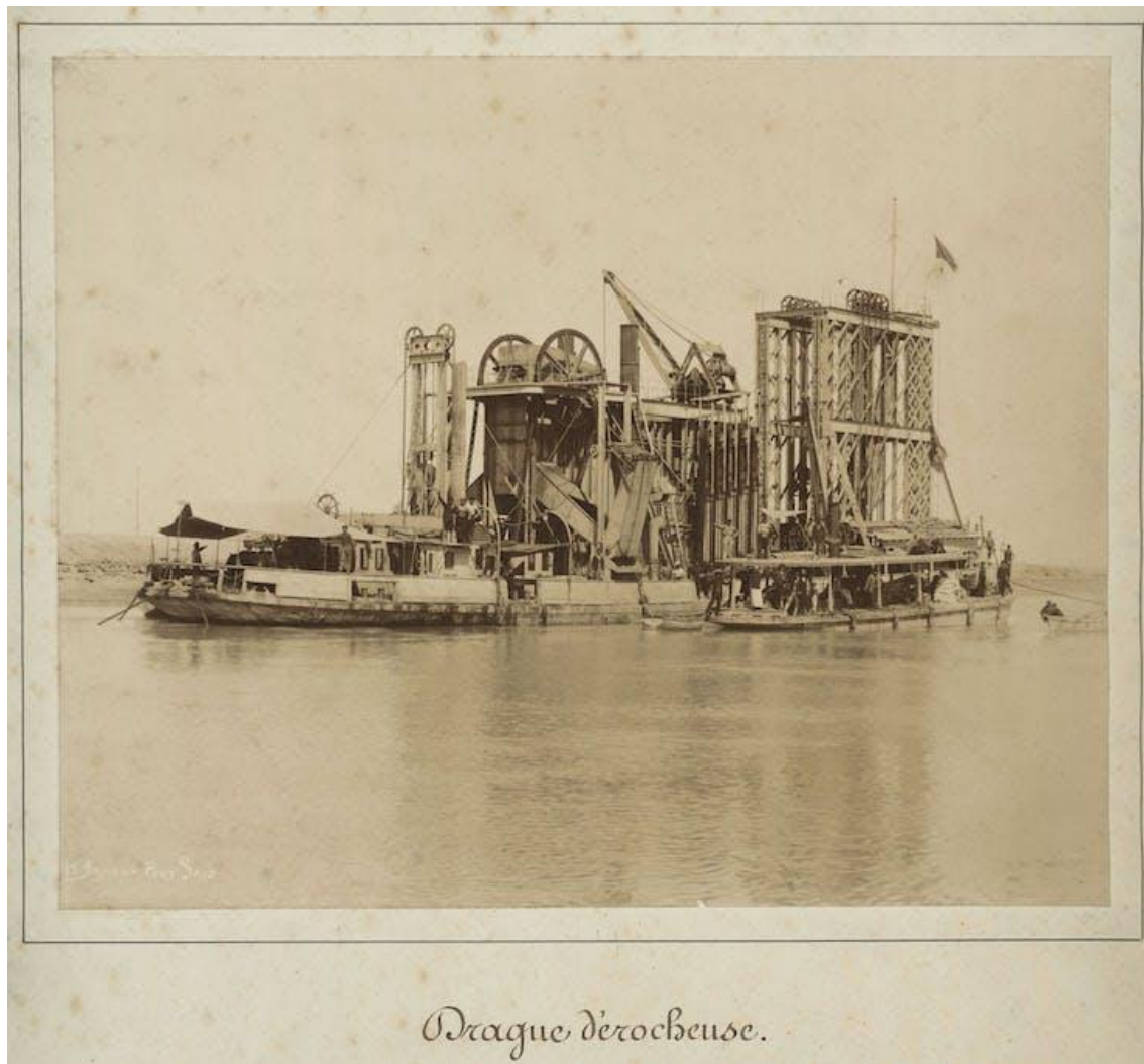
Drague décrocheuse (1869–85), Hippolyte Arnoux and the Zangaki brothers. © Archives nationales du monde du travail (Roubaix)
